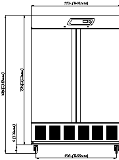
QR(F)-2 FRONT
