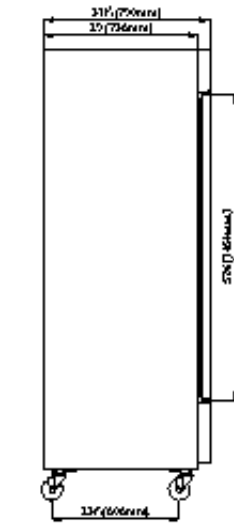
QR(F) SECTION
