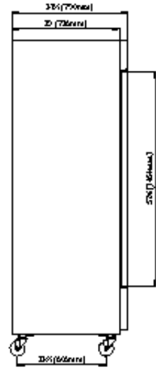
QR(F) SECTION
