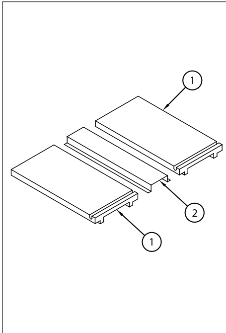
HOT TOP
